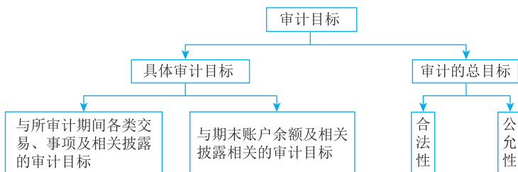
图 1-5 审计目标
