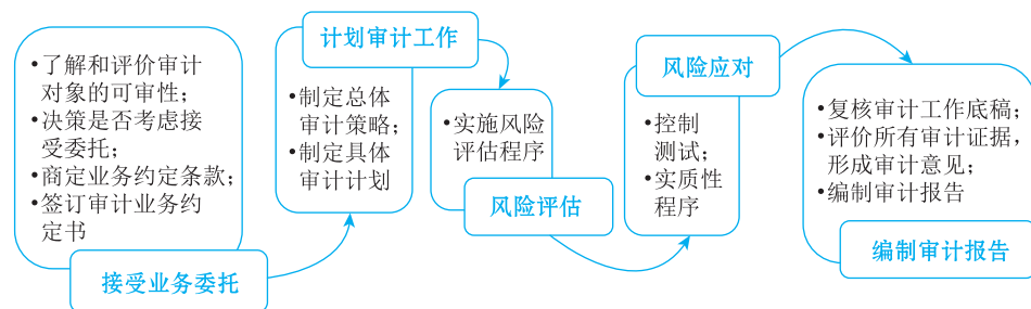
图 1-10 审计过程
